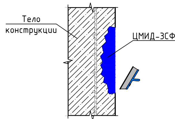
Поз. 5. Нанесение ремонтного состава ЦМИД-ЗСФ
