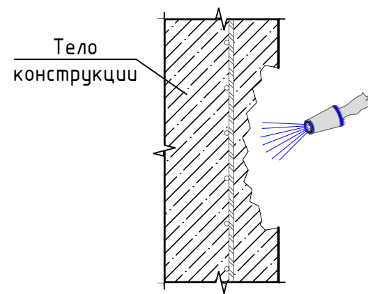
Поз. 4. Очистка и увлажнение поверхности ремонтируемого участка
